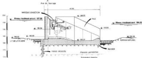
COUPE VERTICALE D'UNE PASSE DE L'OUVRAGE CENTRAL
